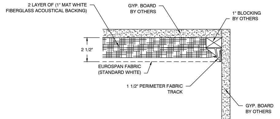
B EDGE AT WALL / SOFFIT WITH BLOCKING 1.5 GYP SCALE: N.T.S.
